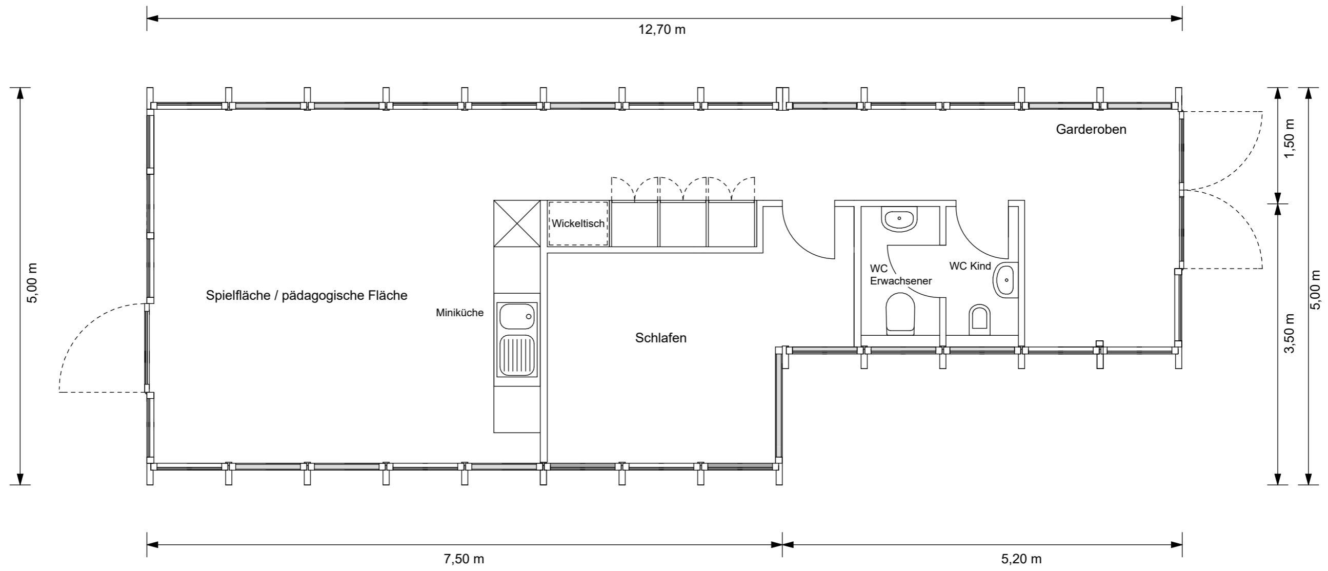
Grundriss
